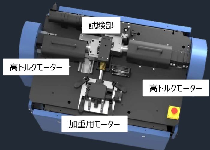
装置構造
